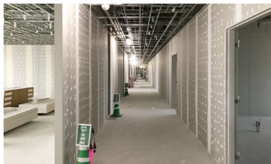
▲ 2階壁・天井施工状況
