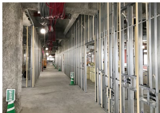
▲ 2階軽量鉄骨壁下地施工状況
