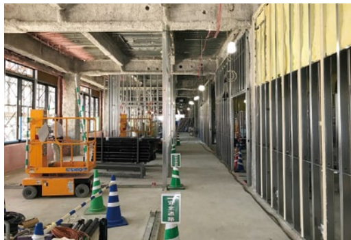
▲ 1階間仕切壁下地施工状況
